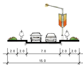
创业路、滨河西路、大岭路道路断面
