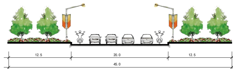
朱东路、县城南外环路西延道路断面
