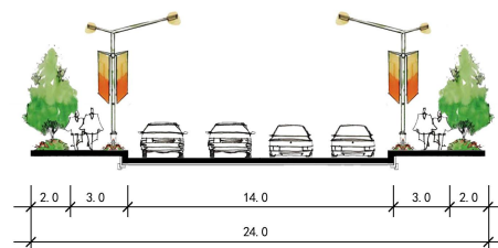
龙查路、府西路、滨河东路、东环路、石沟路、 滨河北路、岭中路道路断面
