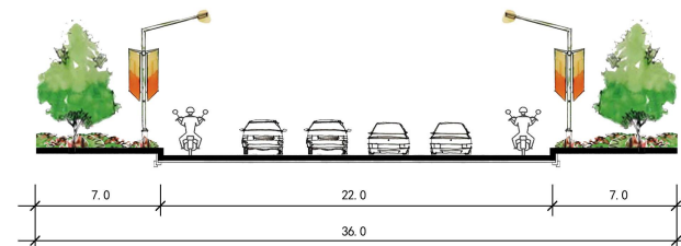
兴郝公路镇区段道路断面
