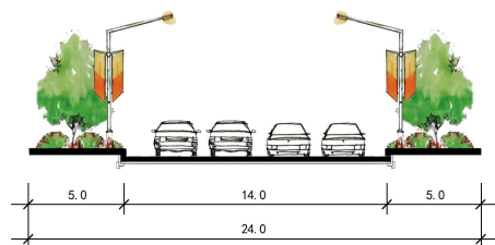
银光路、南二环路、御华路、永安路道路断面
