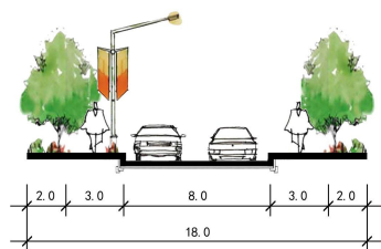
新居路、朱山路道路断面
