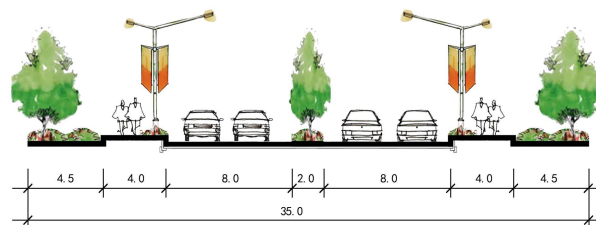
南一环路道路断面
