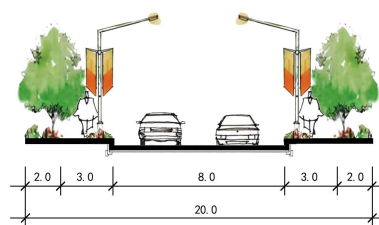
由中路、由东路、北崖路、下庄路、金行路、文化路道路断面
