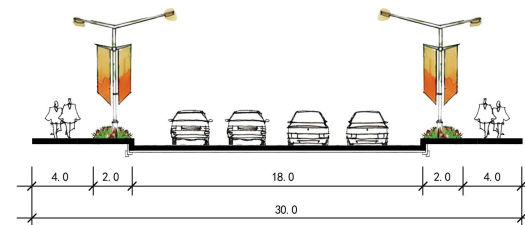
费梁公路镇区段道路断面
