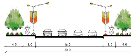
北环路、文涇路（西环路以西、河山路以东）、东环路（文涇路以北）、创业路、天蒙路（向阳路以北、南环路以南）道路断面
