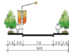
民宿大街道路断面
