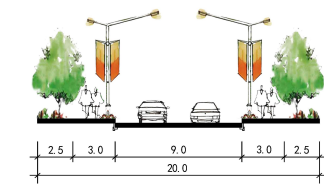
公园路、张庄路、文化路、工业北路、高速北路、工业东路道路断面
