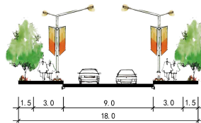
高速南路、永兴路、兴业路、工业西路、旅游路道路断面
