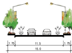
向阳路道路断面
