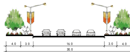
文涇路（西环路—河山路）、工业大道、天蒙路（向阳路—南环路）道路断面
