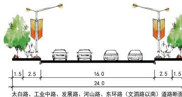
太白路、工业中路、发展路、河山路、东环路（文涇路以南）道路断面
