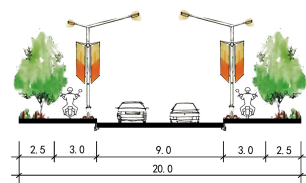
南环路、西环路道路断面
